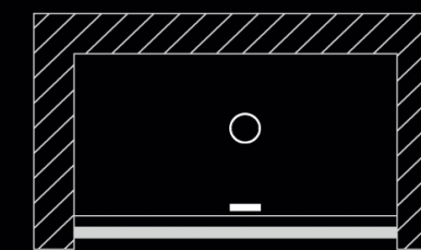
FORMAT Glasverkleidung Version Nische
